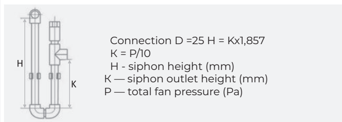
Condensate drain (Fig. 23)
